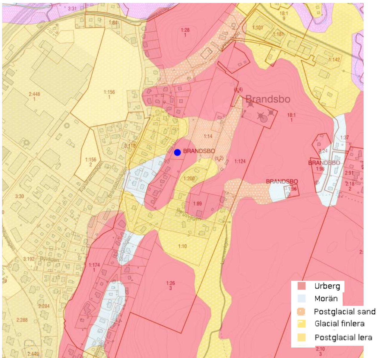
Utsnitt från kommunens samhällsbyggnadskarta över SGU:s jordartsdatalager i området.
